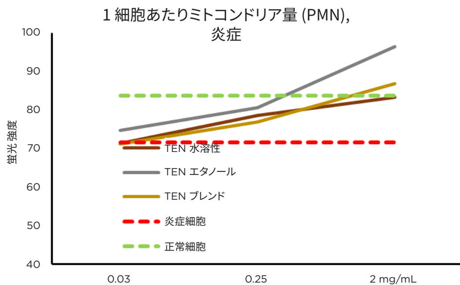
図 20. 多形核細胞 (PMN) あたりのミトコンドリア量は緑色の蛍光強度として示されている。上のグラフは、3重培養の平均標準土標準偏差を示す。未処理細胞 (緑の点線) と炎症細胞 (赤の点線) にデータを施した場合を示す。
