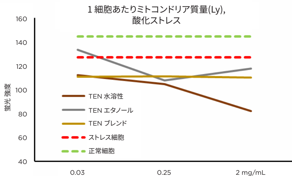
図 15. リンパ細胞あたりのミトコンドリア質量(Ly) は緑色の蛍光強度として示している。上のグラフは、3重培養の平均標準土標準偏差を示す。下のグラフは、未処理細胞 (緑の点線) とストレス細胞 (赤の点線) にデータを施した場合を示す
